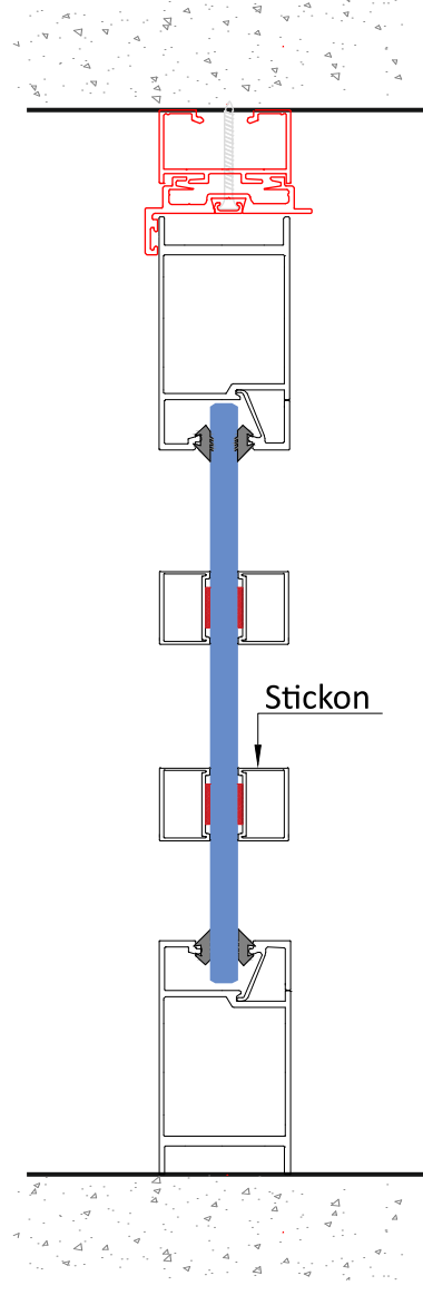
Stick-on Door Configuration
